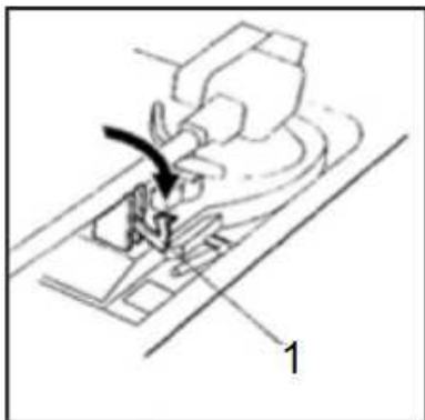
1 = Riegel
